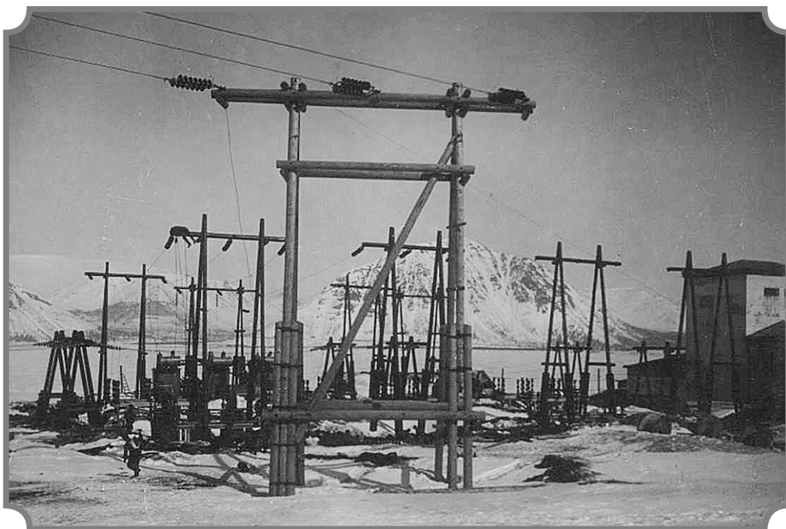
Открытая подстанция № 15 ЦВР «Колэнерго»
